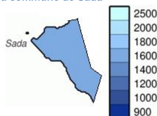
Figure 16 : Cumul de pluie de novembre 2021 à avril 2022 dans la commune de Sada
