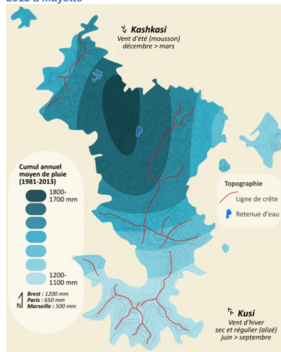
Figure 127 : Pluviométrie moyenne cumulée de 1981 à 2013 à Mayotte
