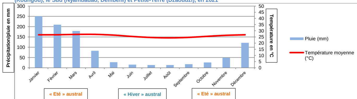
Figure 125 : Diagramme ombrothermique moyenné sur les données du Centre de l'île (Mamoudzou), le Nord (Koungou), le Sud (Nyambadao, Dombéni) et Petite-Terre (Dzaoudzi), en 2021
