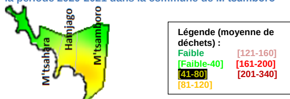
Figure 387 : Densité (lissée) des déchets recensés sur la période 2020-2021 dans la commune de M'tsamboro
