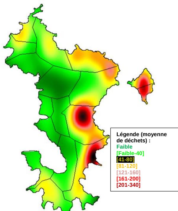
Figure 132 : Densité des déchets recensés dans la nature sur la période 2020-2021 à Mayotte
