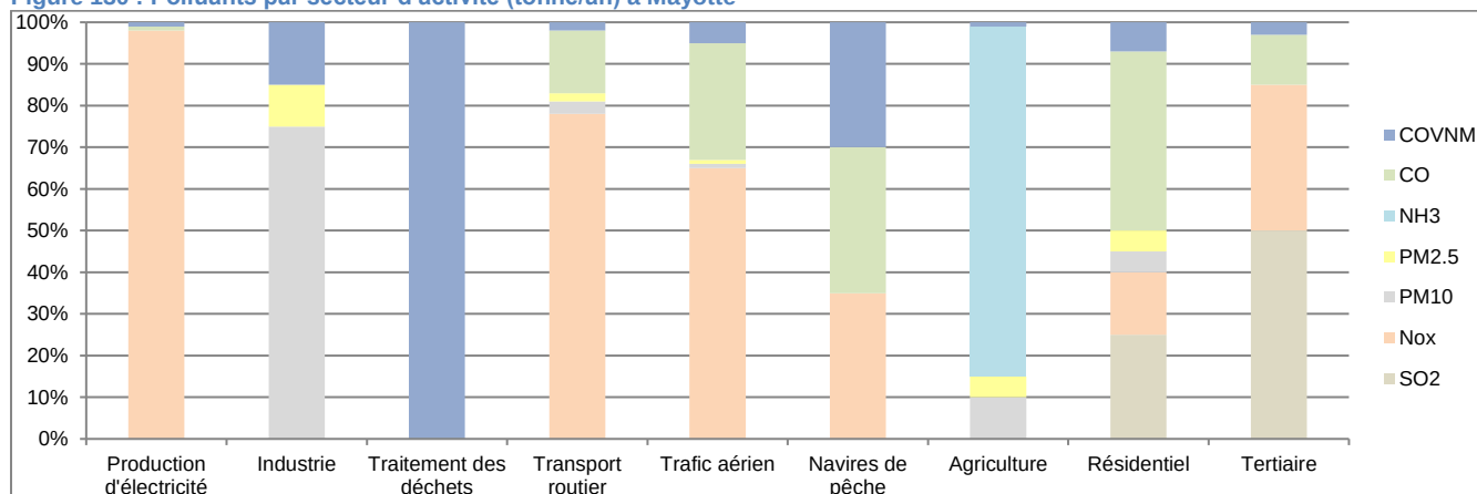
Figure 130 : Polluants par secteur d'activité (tonne/an) à Mayotte
