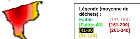
Figure 351 : Densité (lissée) des déchets recensés sur la période 2020-2021 dans la commune de Pamandzi
